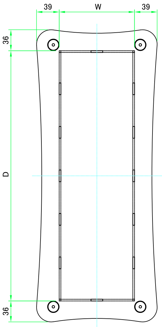
Wパネル1 / W panel 1
