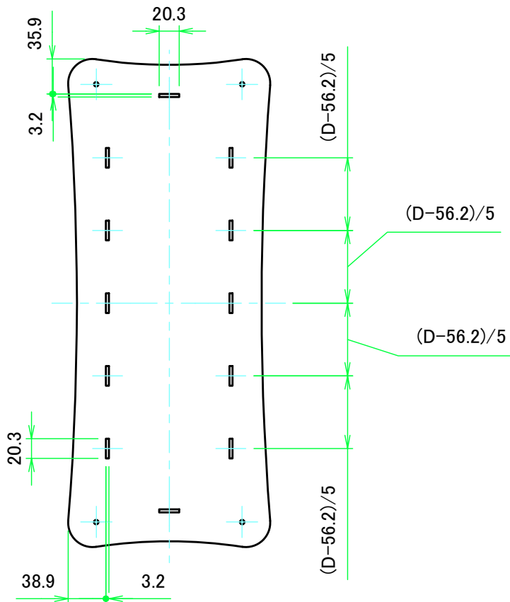
上カバー裏面 / Top cover Backside
